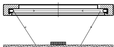
照明示意图
