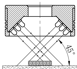
照明示意图
