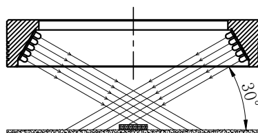
照明示意图
